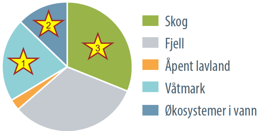
Figur 1. Totalt karbon lagret i norske økosystemer.
